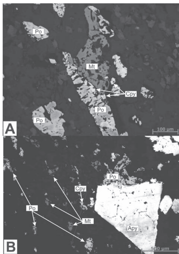
Figura 5 Fotomicrografias (luz refletida, polarizadores paralelos) de BIFs do cinturão metavulcanossedimentar Congonhas-Itaverava com alteração hidrotermal (sulfetação). (A) Zona sulfetada externa, com pirrotita (Po) e calcopirita (Cpy) hidrotermais formando-se a partir de magnetita (Mt). (B) Zona interna de sulfetação, com cristais euédricos a subédricos de arsenopirita (Apy) sobrecrecendo pirrotita e magnetita. A ganga é composta predominantemente por quartzo e carbonatos. Amostras provenientes do furo FVG 24.
