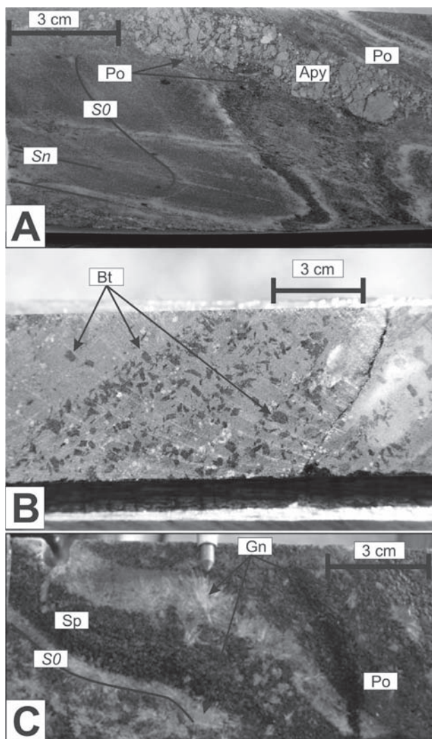
Figura 4 Aspectos da alteração hidrotermal, identificados a partir de testemunhos de sondagem em rochas do Lineamento Congonhas. (A) Veio de quartzo sulfetado, com arsenopirita no núcleo e pirrotita na borda, encaixado em zona de cisalhamento de espessura centimétrica atravessando BIFs. Note a presença de dobra de arraste e lixiviação ao longo de planos da filiação Sn. Furo FVG24. (B) Blastos de biotita hidrotermal crescendo sobre rocha metamáfica da unidade metavulcânica máfica. Furo FIT 02. (C) Crescimento de grunerita em agregados radiais e stibnomelana (lâminas escuras) sobre BIFs da unidade metassedimentar inferior. Furo FCR07. Apy- arsenopirita, Po- pirrotita, Mt- magnetita, S0- laminação sedimentar relicta, Sn- foliação tectônica principal, Gn- grunerita, Sp- stibnomelana, Bt- biotita. Diâmetro dos testemunhos- 6cm; vide Figura 2 para localização dos furos de sondagem.
