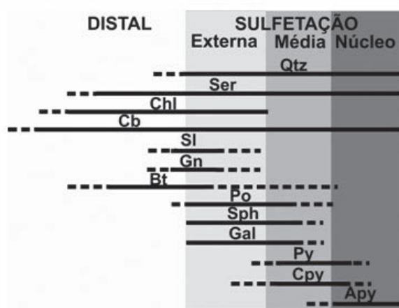
Figura 6 Esquema mostrando as associações de minerais hidrotermais em rochas do CmCI. Ser- sericita, Qtz- quartzo, Chl- clorita, Cb- carbonato, Sl- stilpnomelana, Sph- esfarelita, Gn- grunerita, Gal- galena, Py- pirita, Cpy- calcopirita, Apy- arsenopirita, Po- pirrotita.
