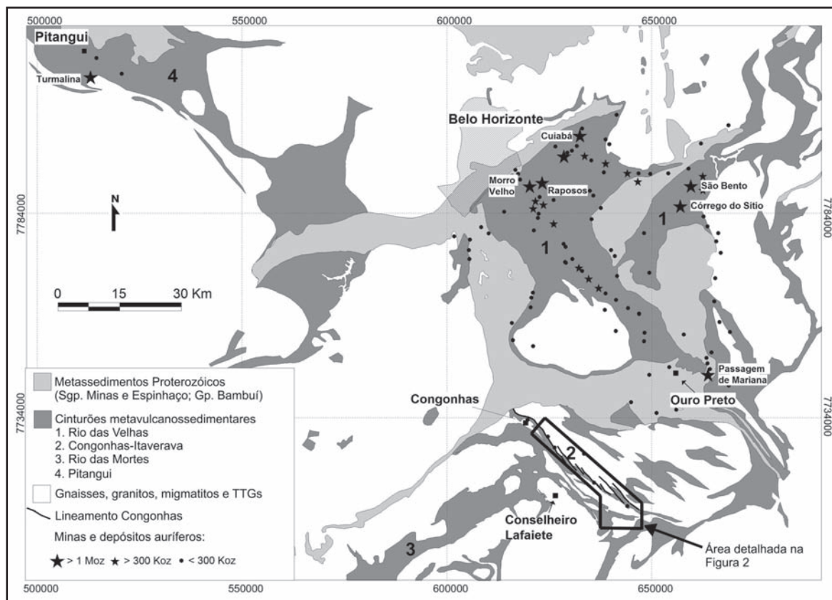
Figura 1 Geologia simplificada do Quadrilátero Ferrífero, com localização do Lineamento Congonhas e do cinturão metavulcanossedimentar Congonhas-Itaverava e dos principais depósitos e ocorrências de ouro, com estimativa de conteúdo metálico. Baseado em Dorr (1969) e interpretações de imagens de levantamento aerogeofísico (K-Th-U CODEMIG). Moz: milhões de onças de Au (dados DNPM).
