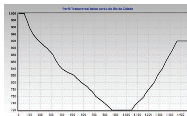
Figura 6 Perfil transversal do baixo curso do rio da Cidade.
