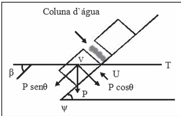
Figura 3 Plano inclinado com a representação das componentes das forças para deslizamento em talude.
