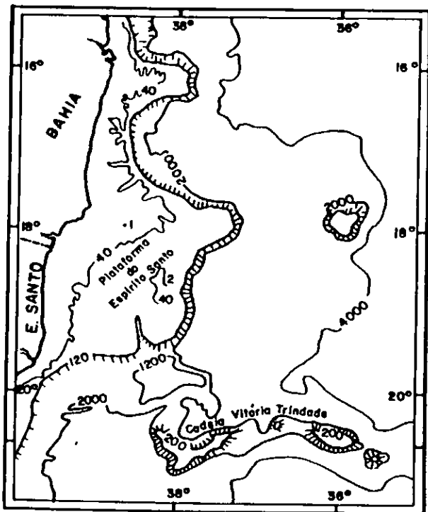
Fig. 1 - Localização da Plataforma do Espírito Santo. Fonte: Brasil. Margem Continental. Mapa batimétrico. Projeto REMAC. 1979.
