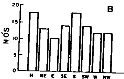
Fig. 2 - Abrolhos: 1956-1983. A) Frequência dos ventos dominantes. B) Intensidade média mensal máxima dos ventos.
