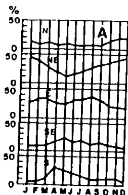
Fig. 2 - Abrolhos: 1956-1983. A) Frequência dos ventos dominantes. B) Intensidade média mensal máxima dos ventos.
