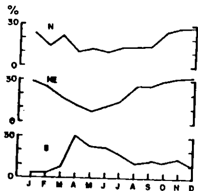
Fig. 2 - Abrolhos: 1956-1983. A) Frequência dos ventos dominantes. B) Intensidade média mensal máxima dos ventos.
