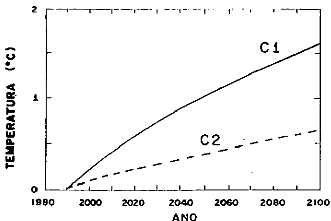
Fig.7 - Aumento da temperatura global calculada a partir dos cenários C1 e C2.
