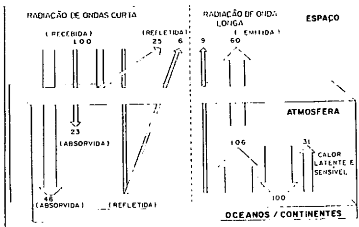
Fig.1 - Balanço de energia no sistema terra-atmosfera.
