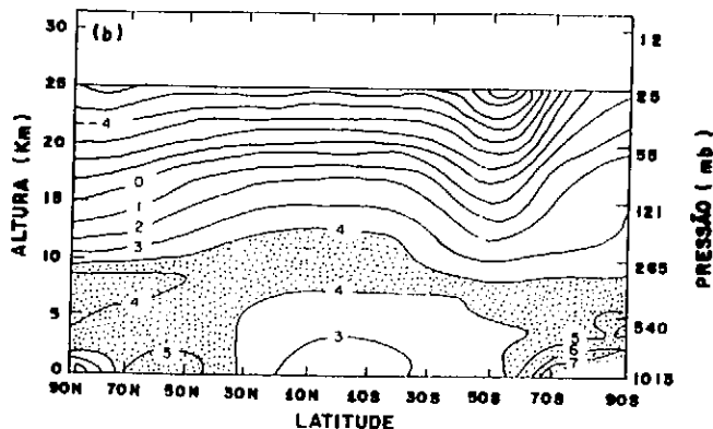
Fig.5 - Variação da Temperatura do ar, média zonal, em função da latitude e da altitude, considerando a duplicação do CO 2 , para junho-julho-agosto, produzido pelo modelo com ajustamento da convecção úmida. (Fonte: Manabe e Weterald, 1988).
