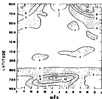
Fig.6 - Variação da Temperatura do ar, média zonal, em função dos meses do ano e da latitude, produzido pelo modelo considerando a duplicação do CO 2 . (Fonte: Schlesinger e Mitchell, 1978).
