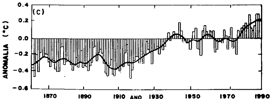
Fig.3 - Variação da temperatura do ar à superfície entre 1850 e 1990. (Fonte: Lindzen, 1990)
