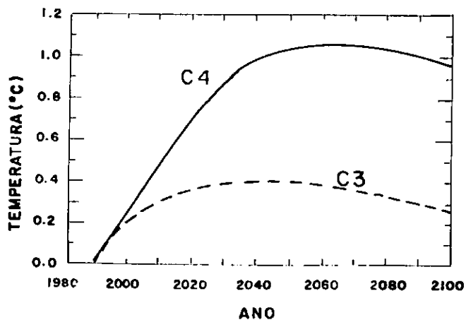
Fig.8 - Variação da temperatura global estimada a partir dos cenários C3 e C4.
