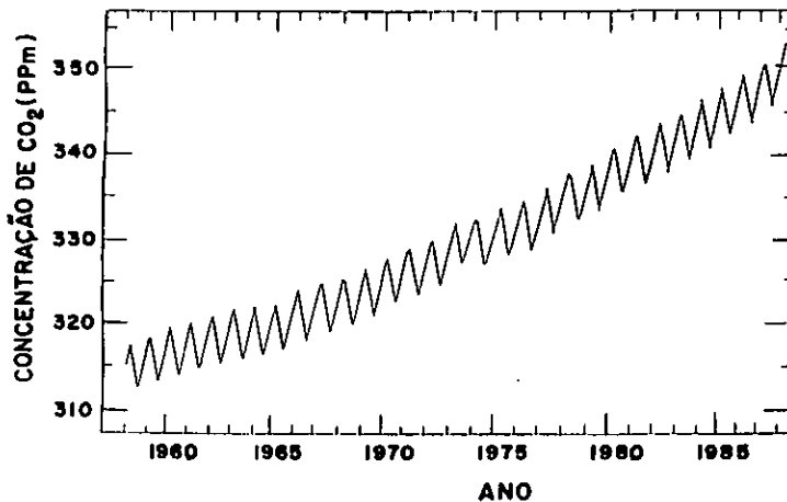
Fig.2 - Variação da concentração do CO 2 em Mauna Loa, Havai. (fonte: Lindzen, 1990).
