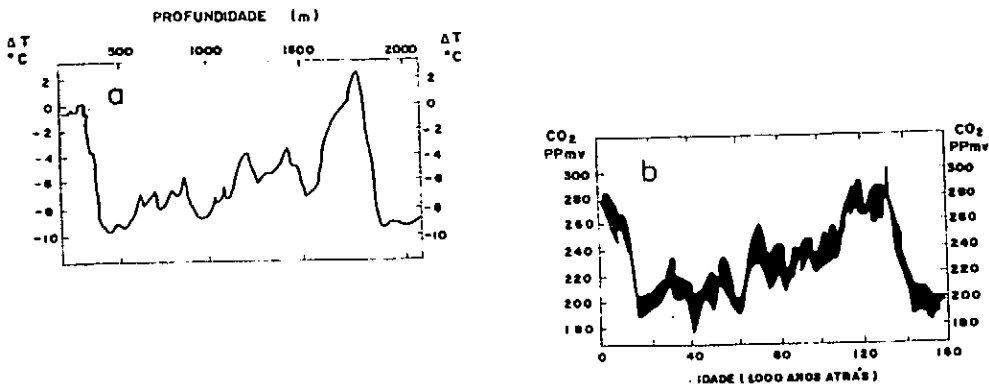
Fig.4 - Variação da temperatura e do conteúdo de CO 2 nos últimos 160.000 anos, determinados a partir do gelo, na base Vostok, Antártida. (Fonte: Houghton et al, 1990)
