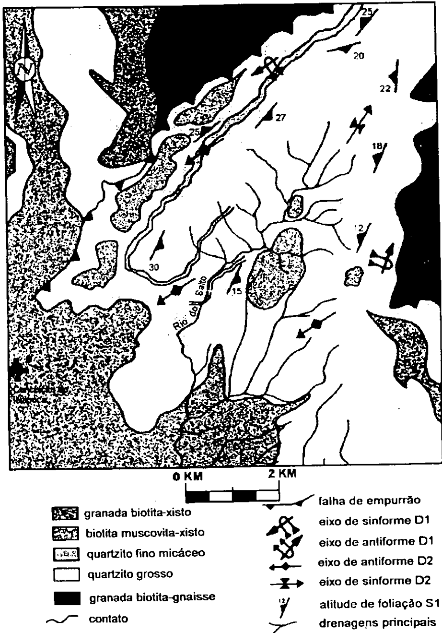
FIGURA 2: Mapa geológico simplificado da Serra do Ibitipoca. Geologia modificada a partir de Nummer (1991)
