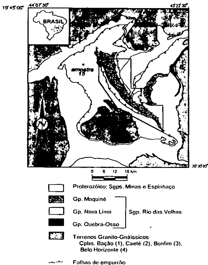
FIGURA 1: Mapa geológico simplificado do Quadrilátero Ferrífero, com localização da área em estudo. Geologia compilada a partir de Dorr II (1969) e Baltazar et al. (1995) Vide texto para detalhes.
