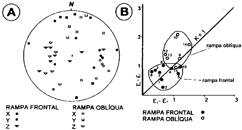
FIGURA 3: (A) Orientação dos eixos dos elipsóides de strain. Diagrama de Schmidt-Lambert, hemisfério inferior. (B) Caracterização do shape fabric. Diagrama logarítmico de Flinn. Vide texto para detalhes
