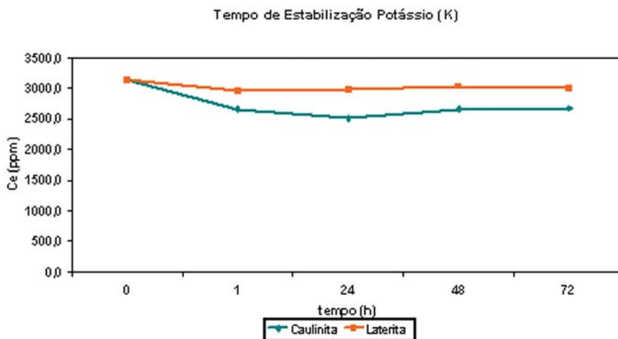
Figura 6 Determinação do tempo de estabilização para o íon potássio (K + ).
