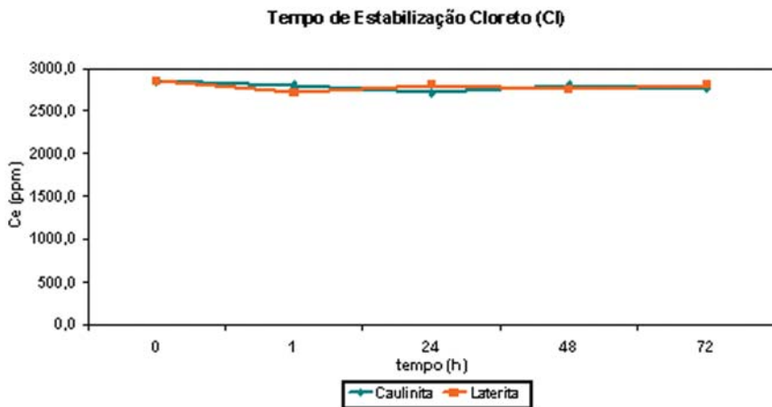
Figura 5 Determinação do tempo de estabilização para o íon cloreto (Cl).
