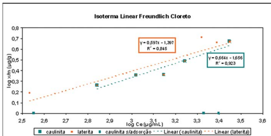
Figura 9 Modelo Freundlich que melhor se ajustou para o cloreto tanto na amostra de solo laterítico quanto para a do material caulinitico.
