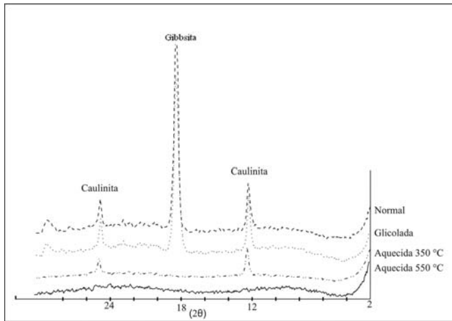
Figura 4 Difratograma referente a fração argila desferrificada da amostra de solo laterítico
