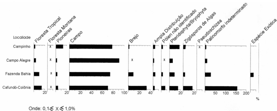
Figura 2 Diagrama palinológico, apresentando as percentagens totais dos diferentes grupos ecológicos encontrados nas localidades analisadas.
