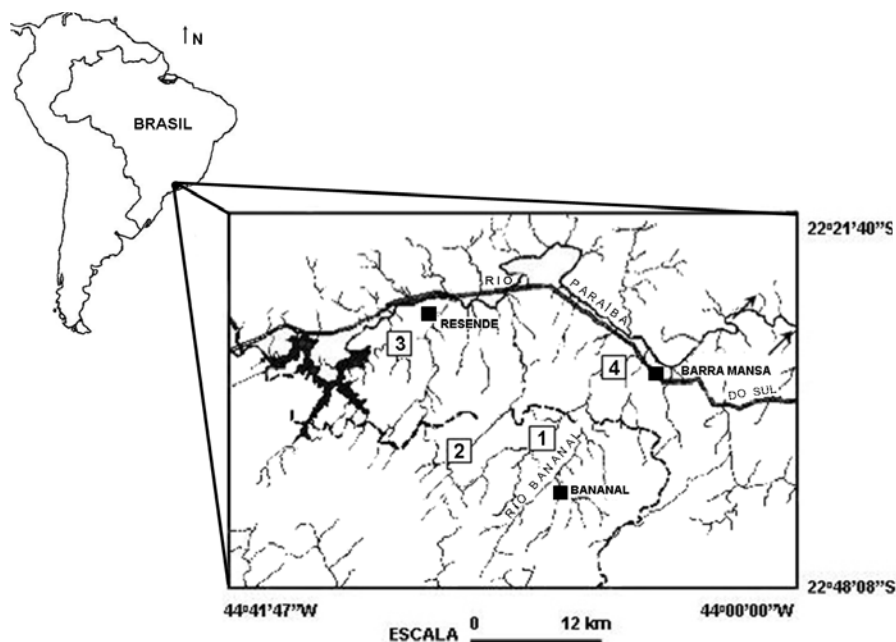
Figura 1 Mapa de localização, destacando-se a região estudada (modificação de Barros et al. , 2000).
