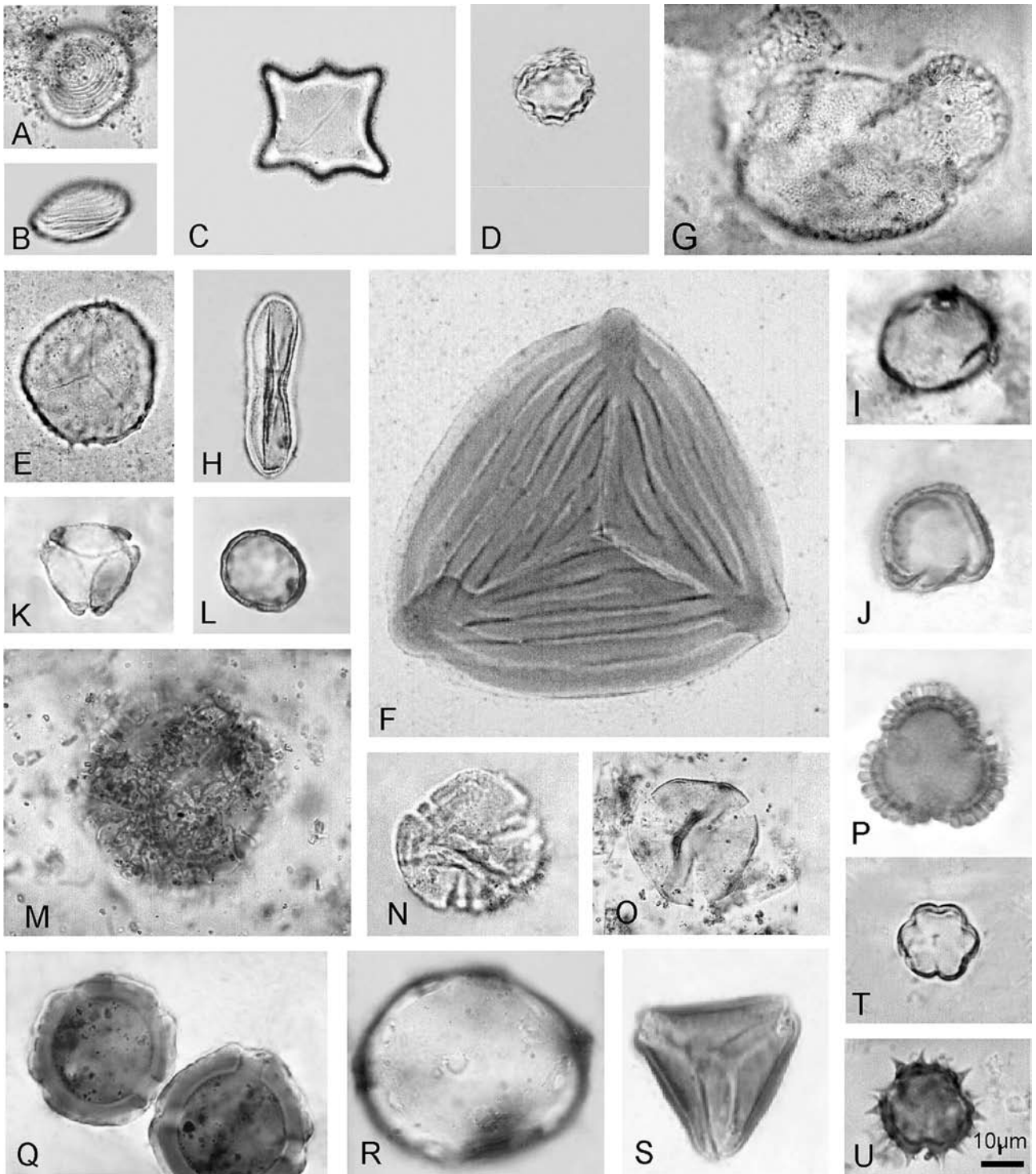
Figura 4 Fotomicrografias de tipos polínicos significativos observados (A e B) Incertae sedis : Pseudoschizaea; (C) Algae, Zygnemataceae: Mougeotia; (D) Algae: Zygnemataceae, Zygnema ; (E) Bryophyta, Phaeoceros; (F) Pteridophyta, Schizaeaceae: Anemia ; (G) Podocarpaceae: Podocarpus ; (H) Apiaceae: Eryngium ; (I) Poaceae; (J) Eriocaulaceae: Paepalanthus ; (K) Mytaceae: Myrcia ; (L) Chenopodiaceae; (M) Winteraceae: Drymis ; (N) Euphorbiaceae: Alchornea; (O) Bignoniaceae; (P) Aquifoliaceae: Ilex ; (Q) Malpighiaceae: Tetrapteris ; (R) Apocynaceae; (S) Loranthaceae: Struthanthus ; (T) Melastomataceae/Combretaceae; (U) Asteraceae.
