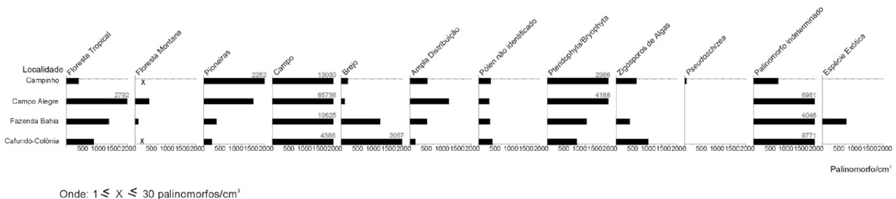
Figura 3 Diagrama palinológico, apresentando a concentração total (palinormorf/cm 3 ) dos diferentes grupos ecológicos encontrados nas localidades analisadas.
